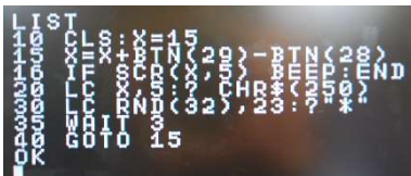
写真 2 BASIC のプログラム
