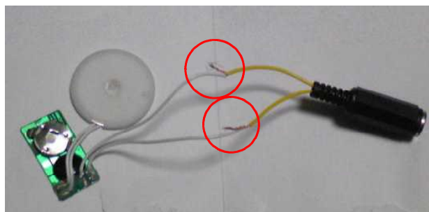
⑤ジャックをつなぐ
