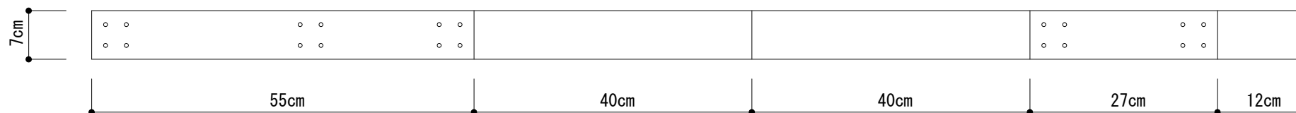
足板 2 枚 (厚さ1.6cm)
